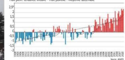
Evolution des températures annuelles dans les Alpes françaises entre 1900 et 2020
